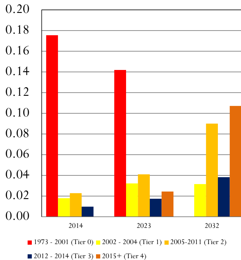
VOC (TPD)
